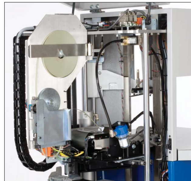
Leichter Zugriff zum Papierrollen Wechsel und Wartung.
